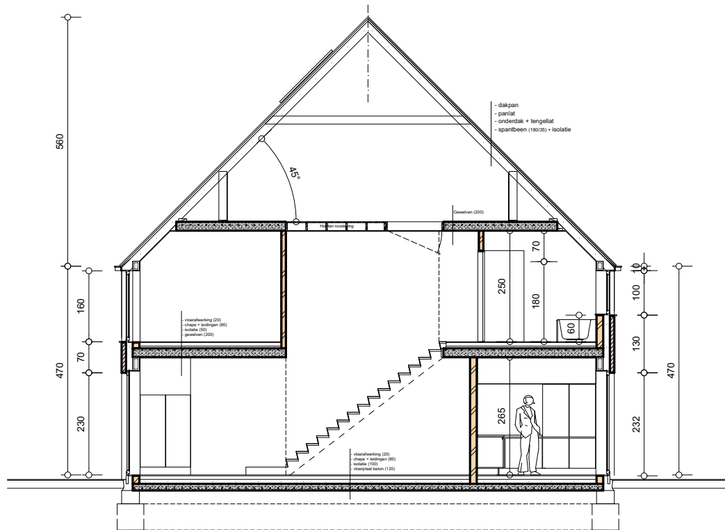
- Langsdoorsnede -
