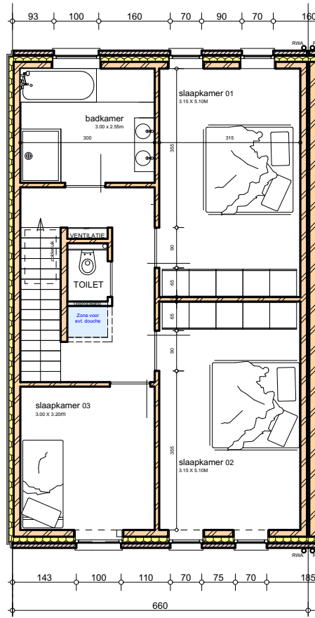
Verdieping
